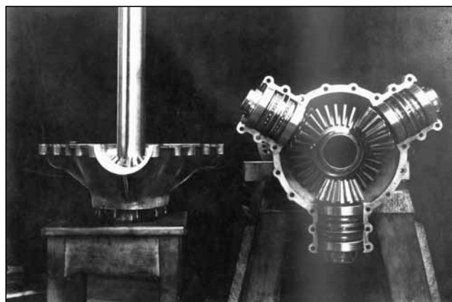
Demontovaná převodová skříň vrtulníku Ing. Viléma Žurovce. Vlevo v bočním pohledu je dolní část skříňe s hřídelí horního rotoru. Vpravo pohled na průřez horní částí převodové skříňe s hřídelí dolního rotoru.
