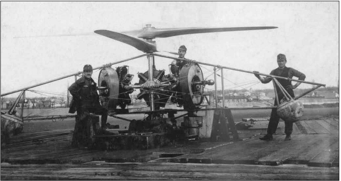
Obsluha připravuje vrtulník ke startu. Stroj je umístěn na přistávacím vaku. Jsou patrný tři hvězdicové motory, před nimi jsou upevněny plechové palivové nádrže vejčitého tvaru. Vrtulník na této fotografii nemá pozorovací gondolu.
